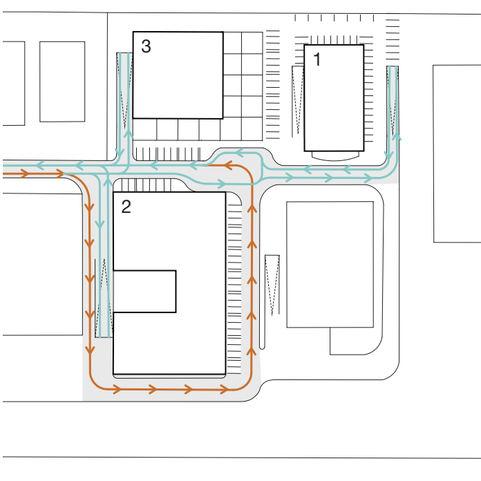
FAZA 2 - zgrajen objekt DCB III in DCB II - dovodne poti za tovorna vozila vodijo okoli objekta DCB II - brez tovornih pred DCB I
