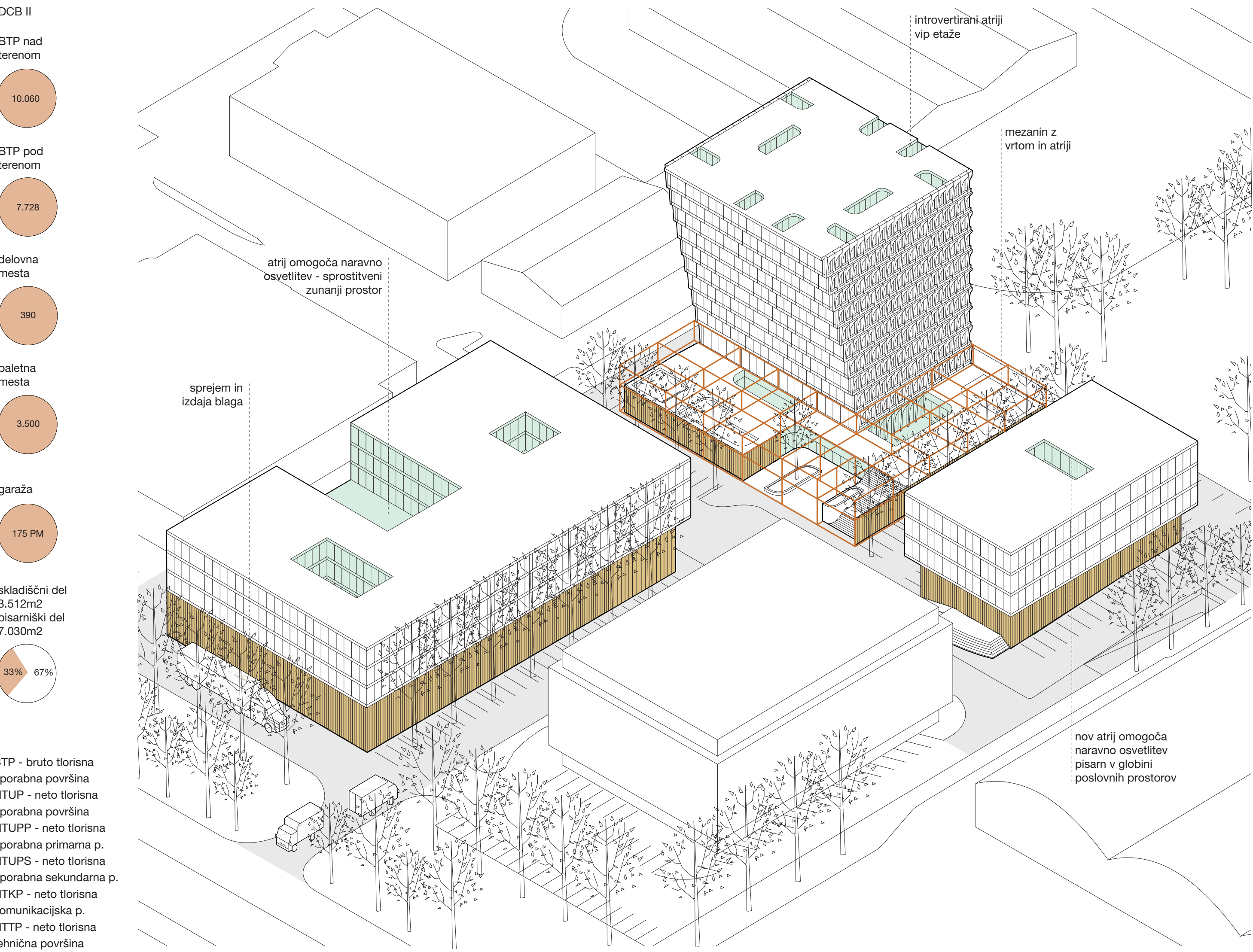
AKSONOMETRIJA OBMOČJA POSLOVNEGA KOMPLEKSA DCB 1:500
