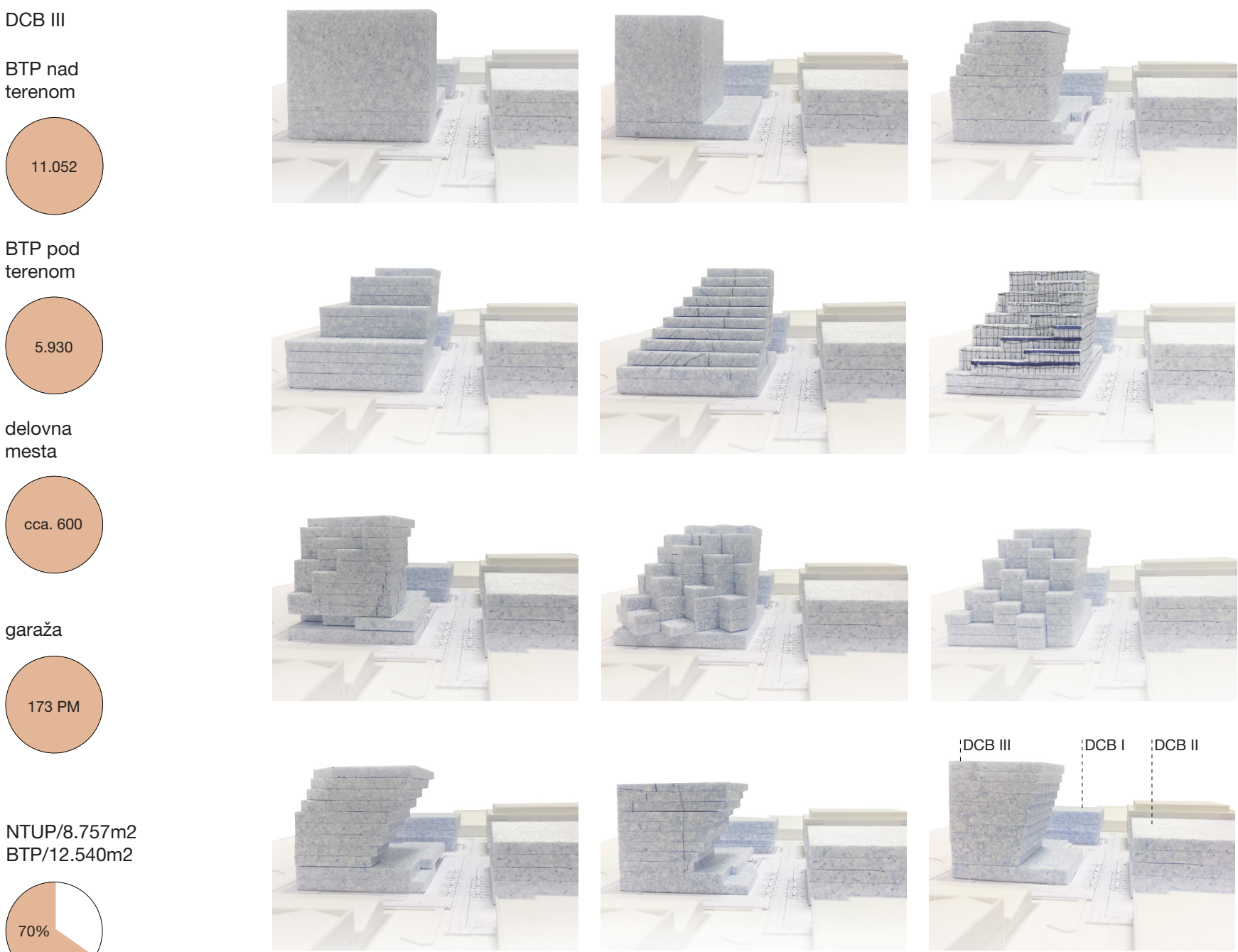
VOLUMETRIČNA ŠTUDIJA OBJEKTA DCB III IZ SMERI GLAVNEGA DOSTOPA Z LESKOŠKOVE CESTE Stolp stavbe DCB III, ki se stopničasto širi z mezanina proti vrhu deluje skupaj s stavbo DCB II in DCB I kot okvir, ki prostorsko poudari atmosfero in aktivnosti v podiju in na mezaninu.
