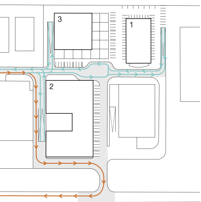
FAZA 3 - zgrajen objekt DCB III in DCB II - dovodne poti za tovorna vozila se vodijo po robu parcele DCB II in do Letališke ceste (po izgradnji novega priključka) - v območju med zgradbami brez tovornega prometa
