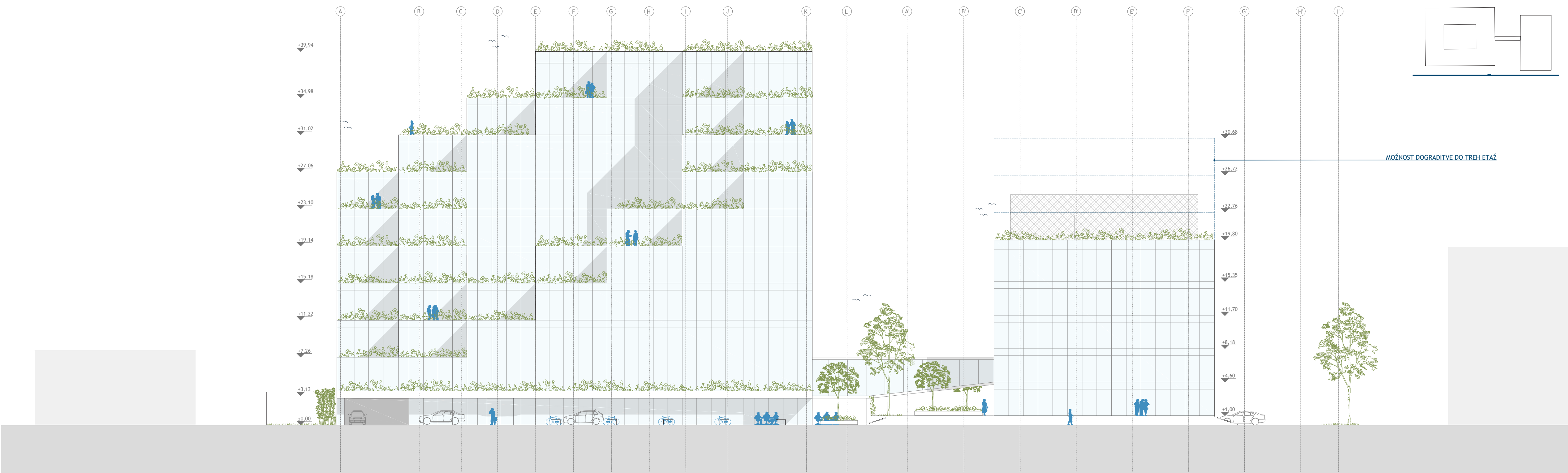
JUŽNA FASADA m 1:250
