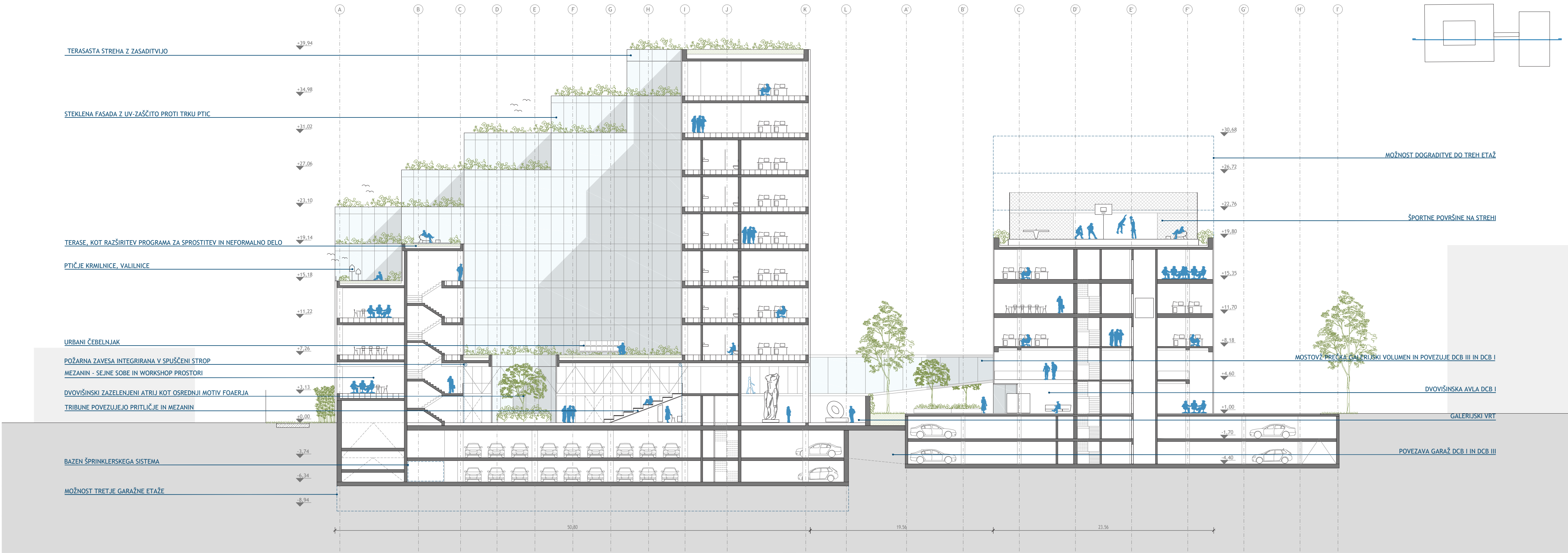
VZDOLŽNI PREREZ ČEZ OBJEKTE DCB III IN DCB I
