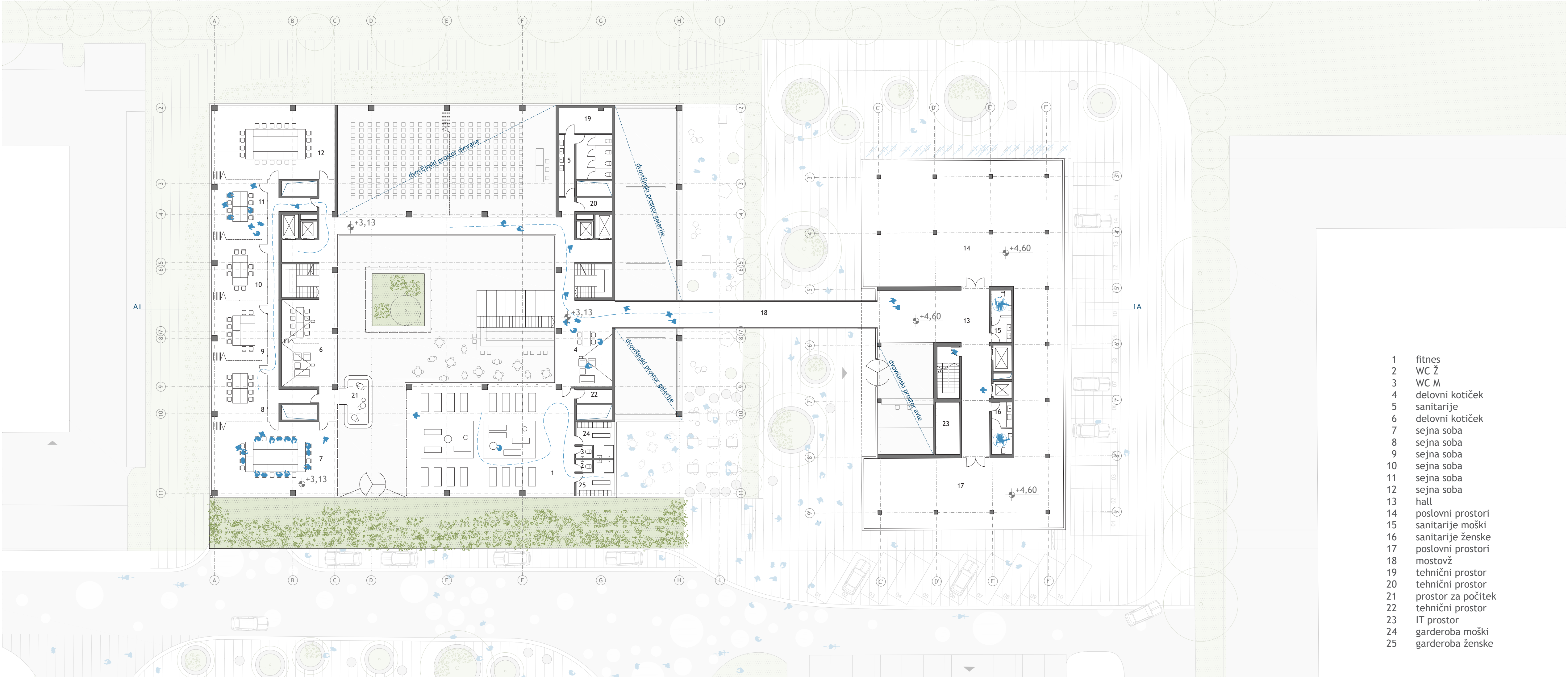
TLORIS MEZANINA m 1:250
