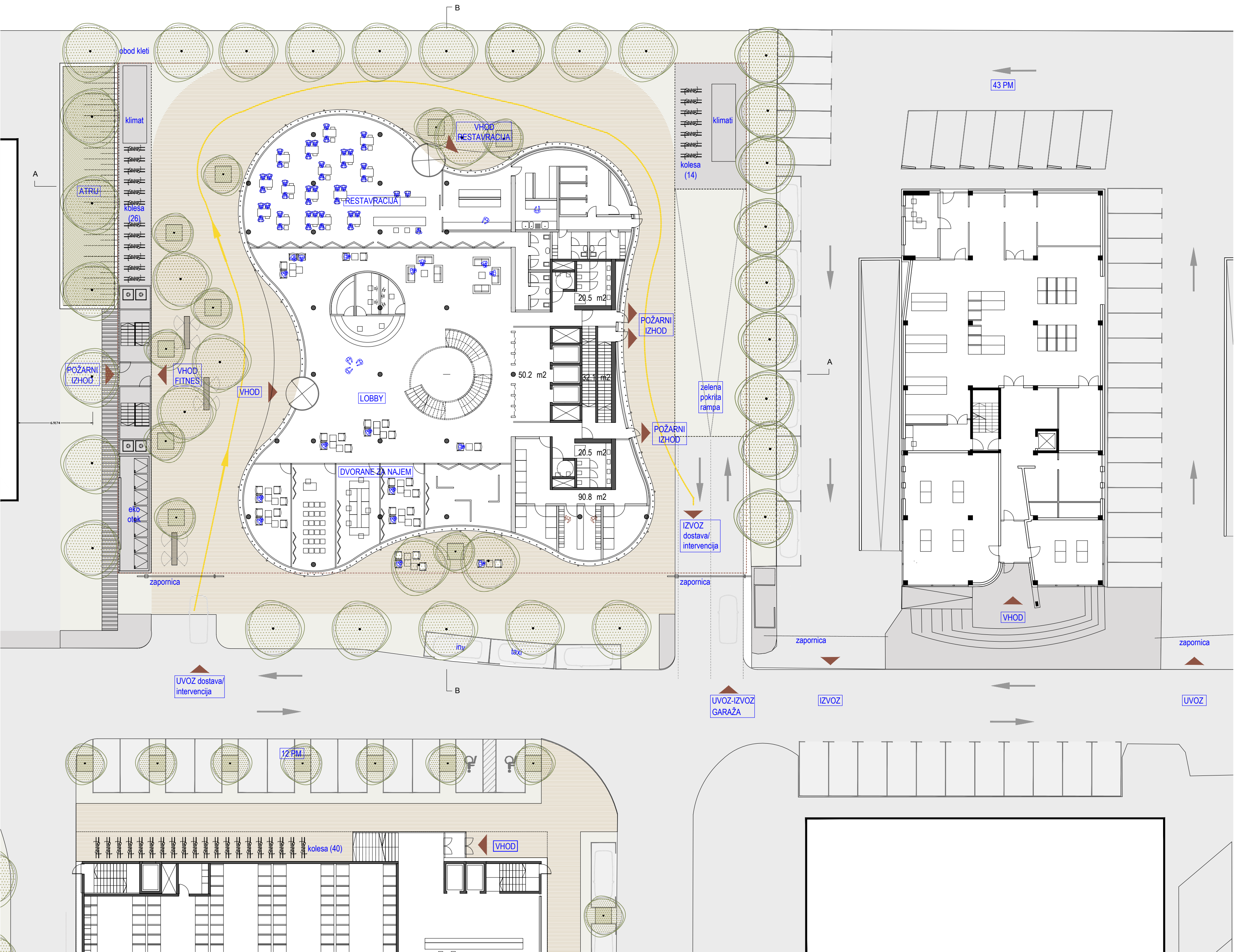
TLORIS PRITLIČJA 1:250
