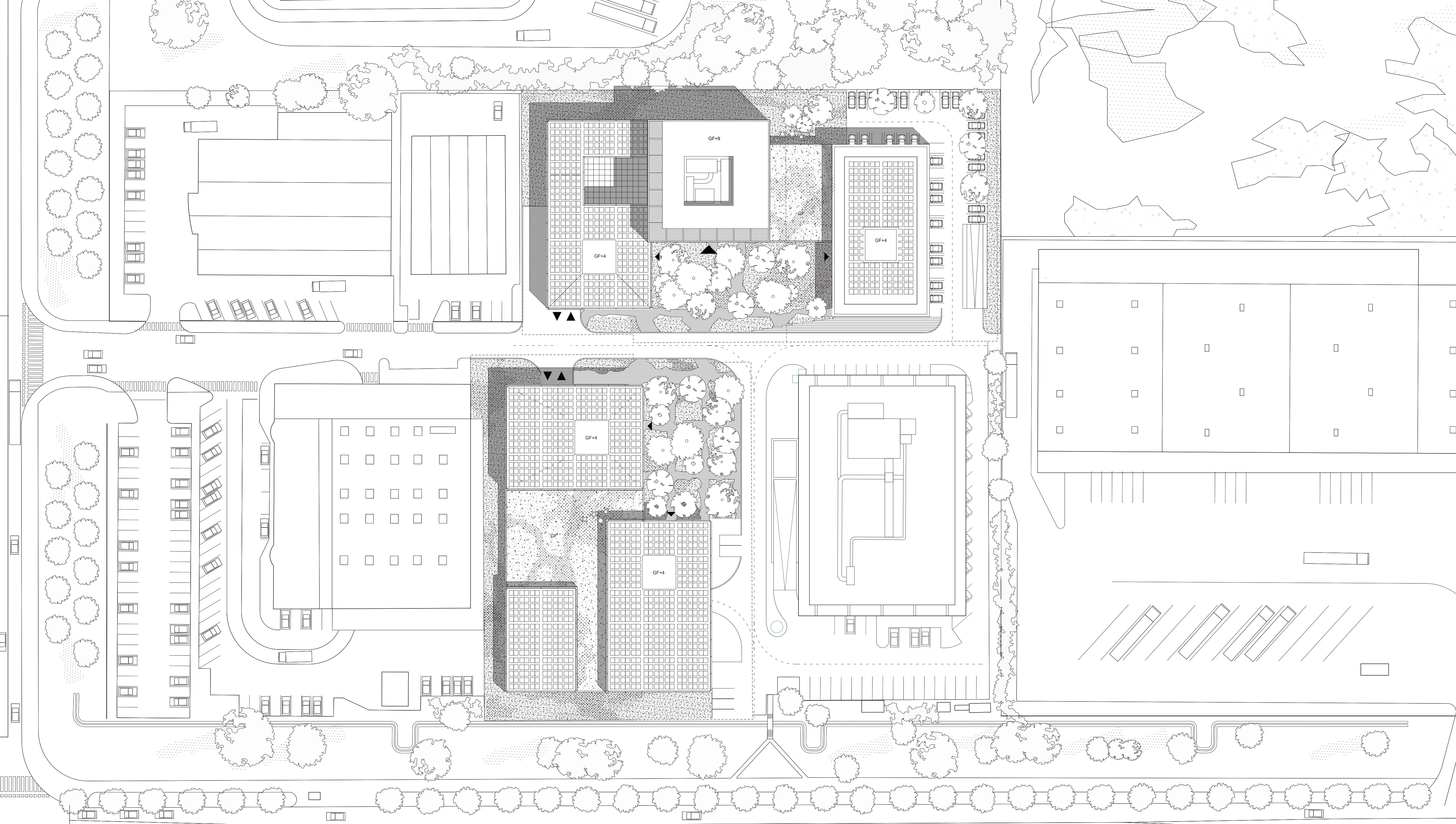
Site plan 1:500
